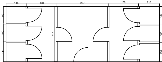
Sanitariaty dla dziewczyn - stan obecny
