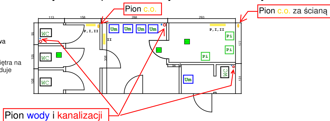
Sanitariaty dla chłopców i nauczycieli - stan obecny
