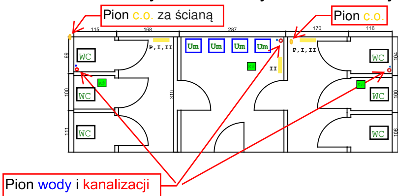
Sanitariaty dla dziewczyn - stan obecny
